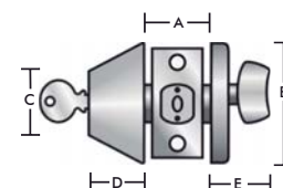
Cerrojo de Seguridad Mod. CS 1 MC
