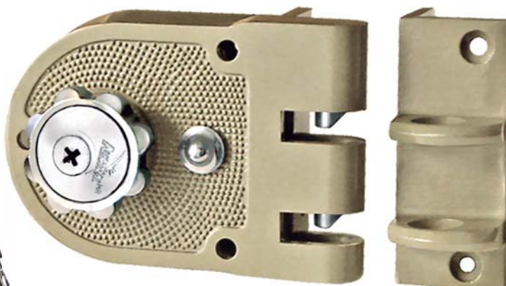
Cilindro exterior integrado a la cerradura
